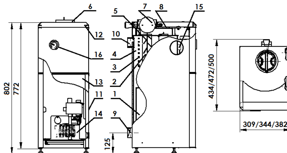
Рис.1. Котлы КСЦ-Г/ГВ-10/12/16...
